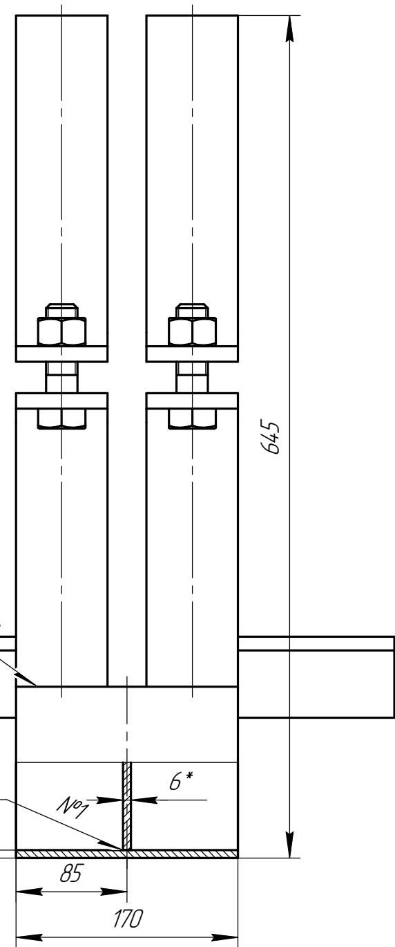
Дет. поз. 4 (1:2,5)
