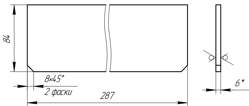
Дет. поз. 2 (1:2,5)
