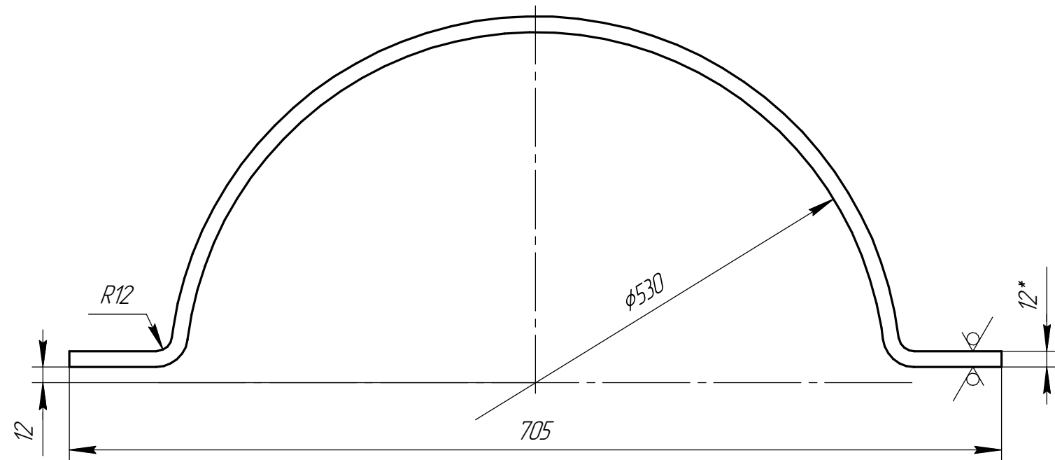
Дет. поз. 3
